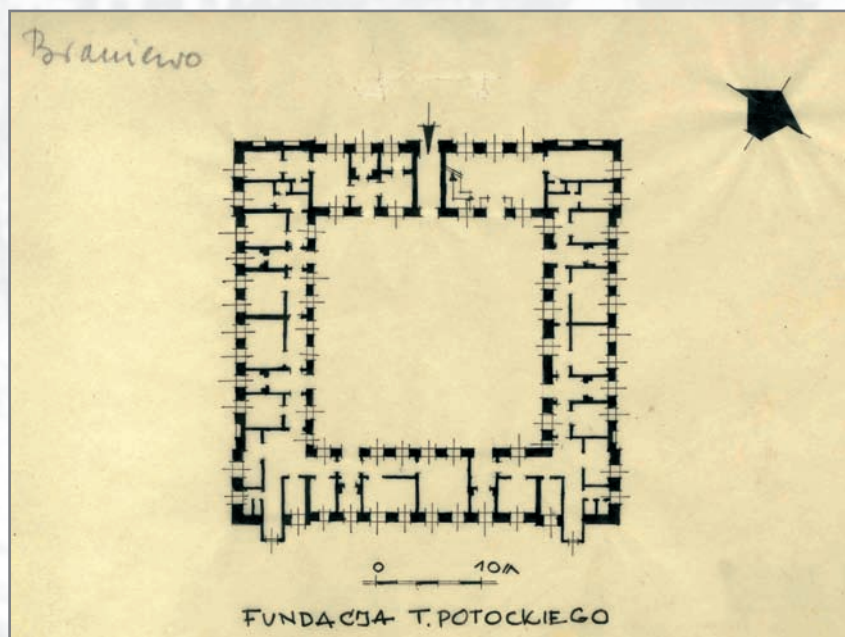
Rzut przyziemia założenia domu dla konwertytów w pocz. XVIII wieku
